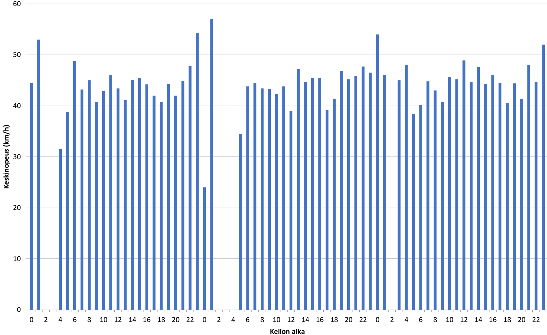
Keskinopeus - 7.11.2023-9.11.2023 - Piste 2 suunta A
