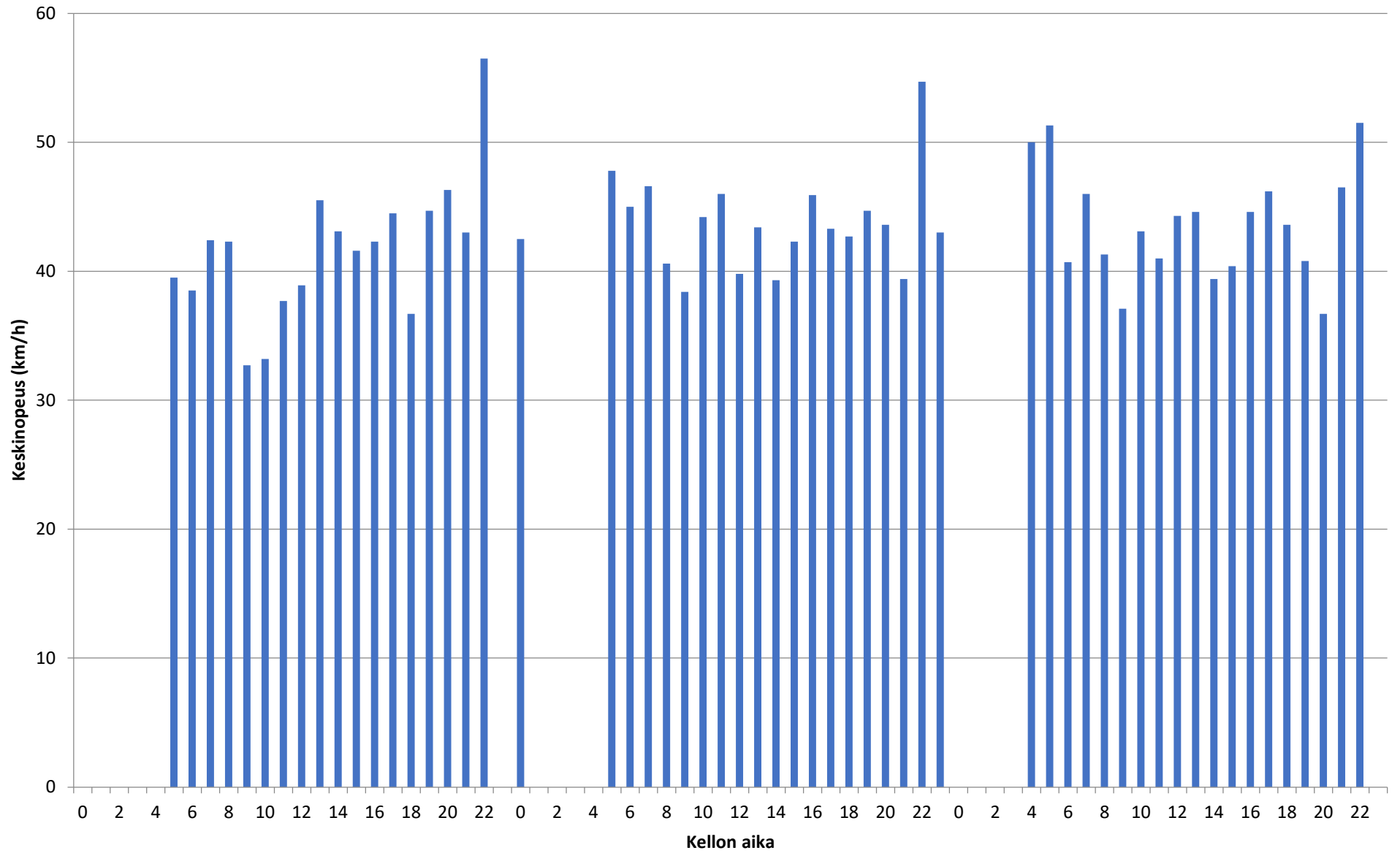
Keskinopeus - 7.11.2023-9.11.2023 - Piste 1 suunta B
