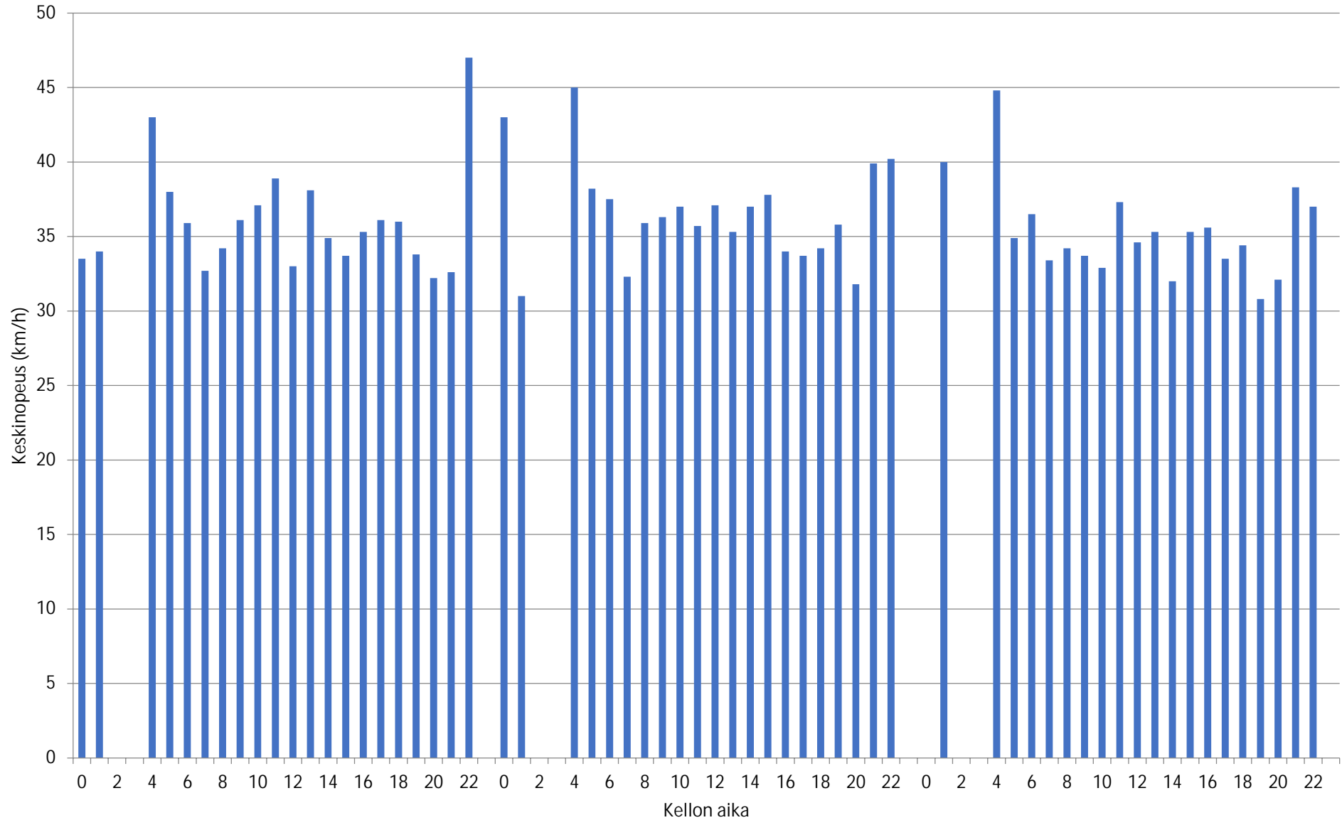
Keskinopeus - 7.11.2023-9.11.2023 - Piste 5 suunta A
