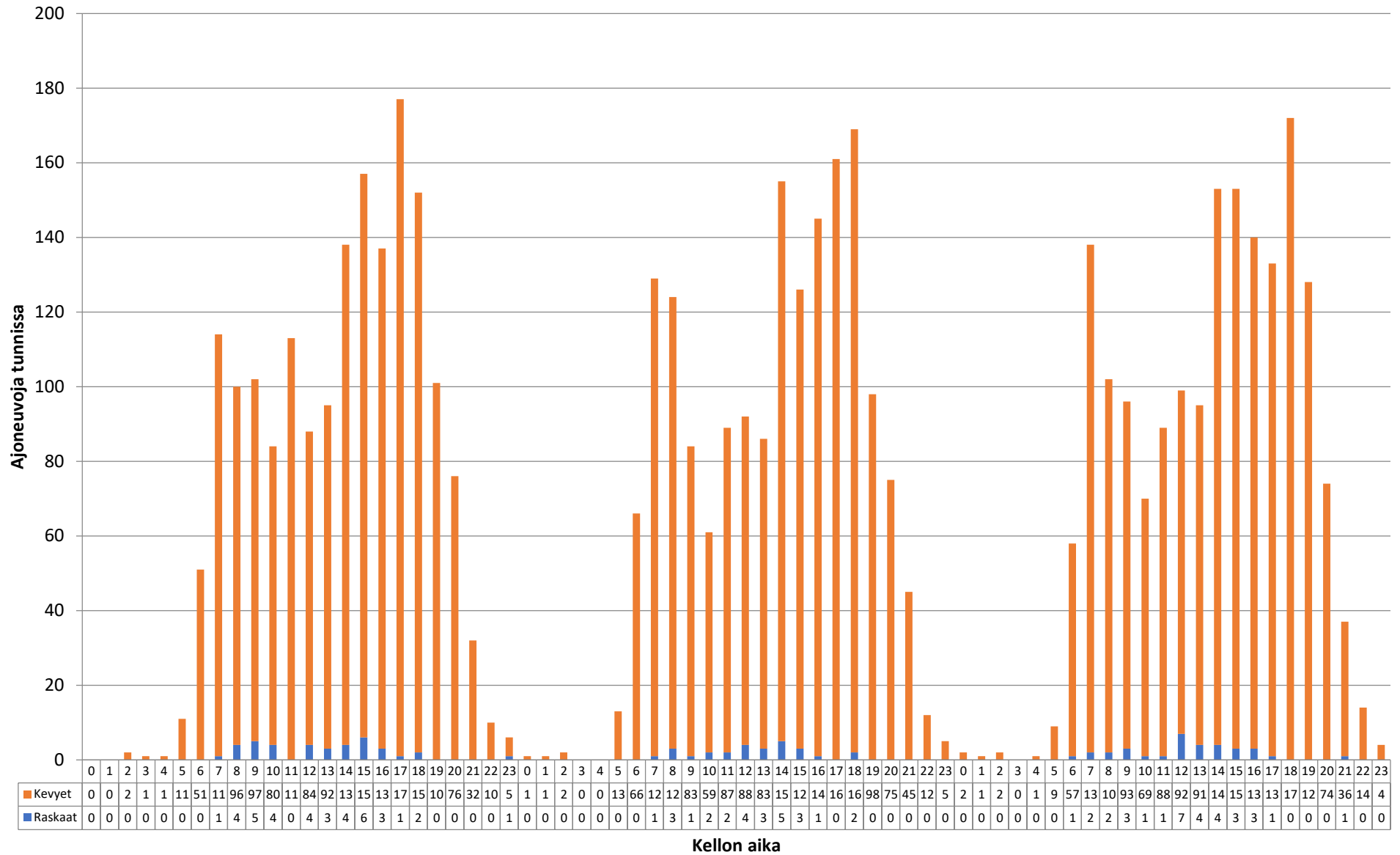
Liikennetiedot ajoneuvoryhmittäin - 7.11.2023-9.11.2023 - Piste 3 suunta B
