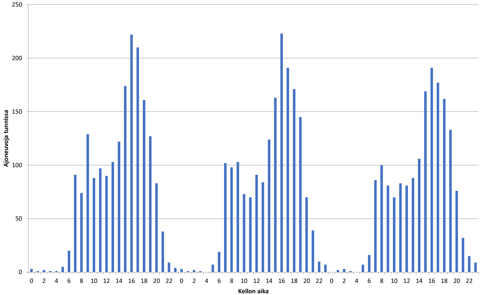
Liikennetiedot - 7.11.2023-9.11.2023 - Piste 3 suunta A
