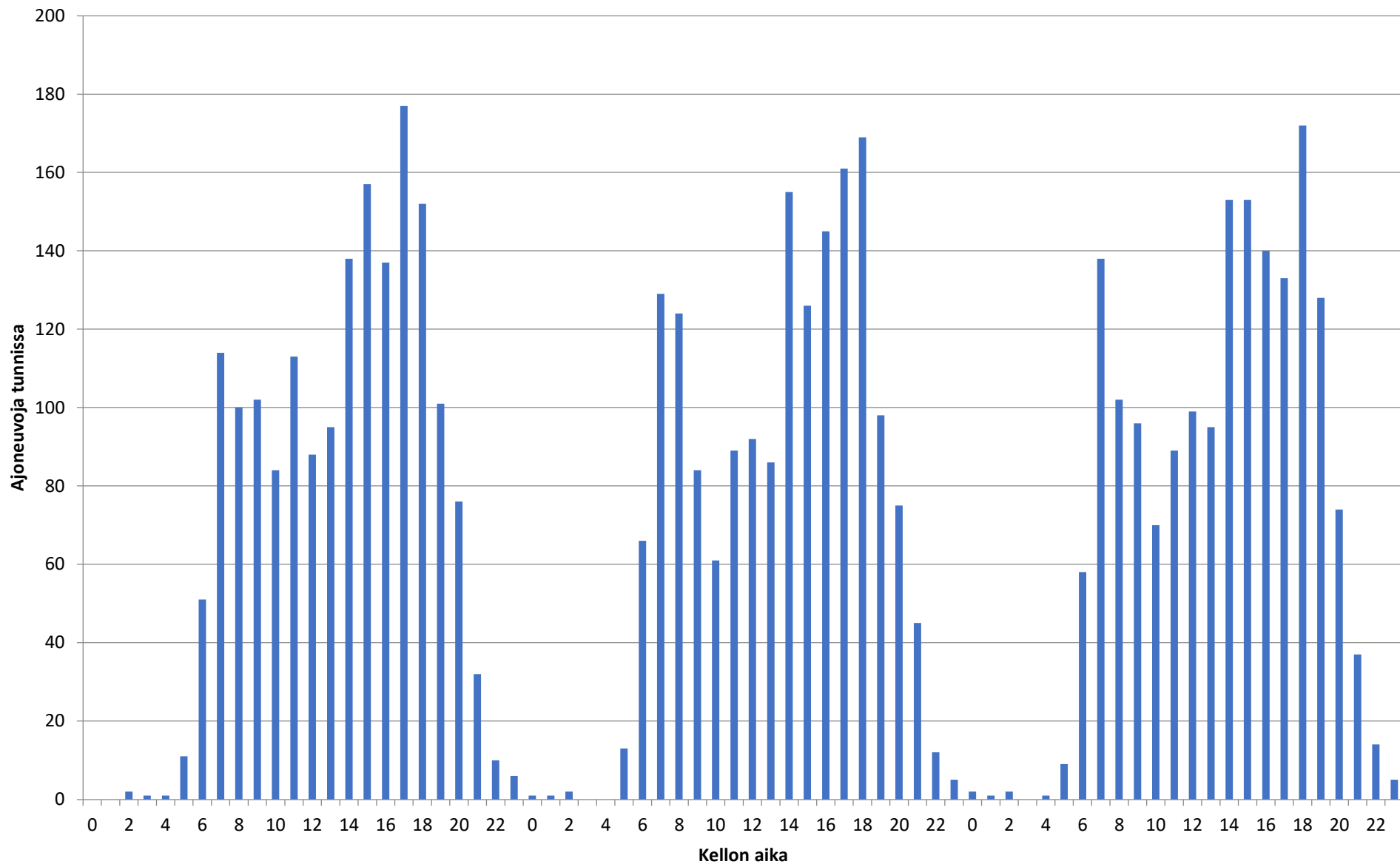
Liikennetiedot - 7.11.2023-9.11.2023 - Piste 3 suunta B
