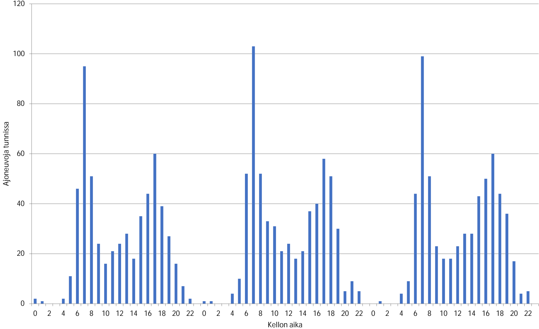
Liikennetiedot - 7.11.2023-9.11.2023 - Piste 5 suunta A
