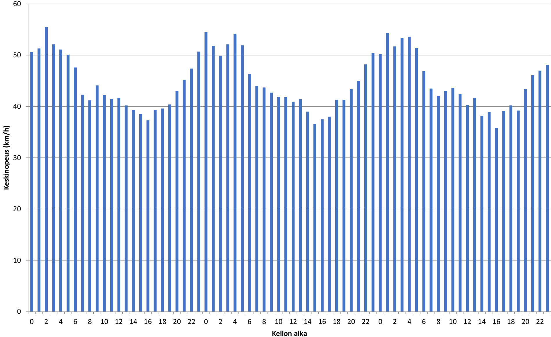
Keskinopeus - 7.11.2023-9.11.2023 - Piste 4 suunta A
