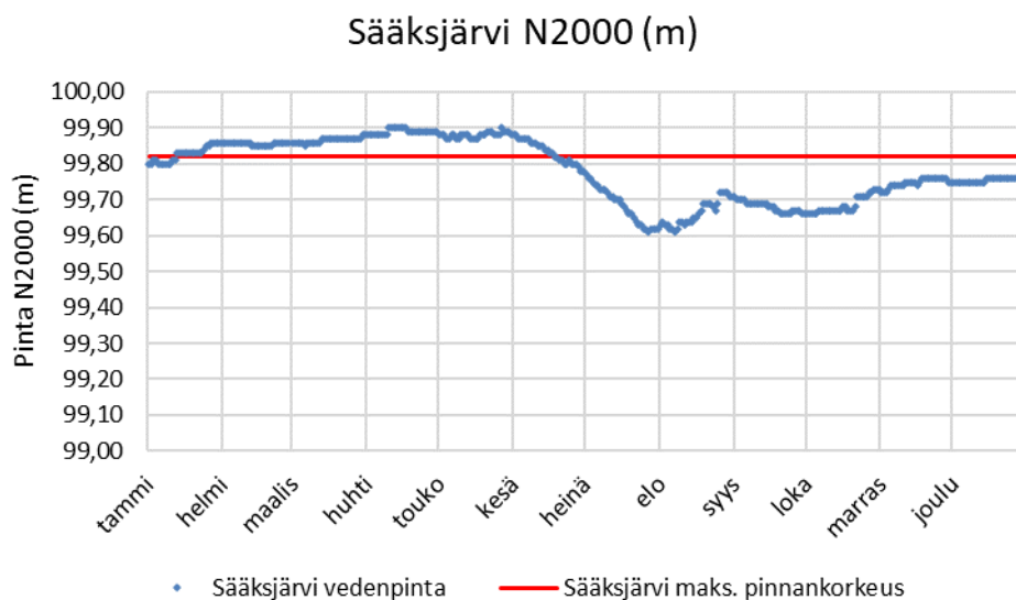
Kuva 7.1. Sääksjärven vedenkorkeus N2000-järjestelmässä vuonna 2021. Lisäveden juoksutus Sääksjärveen on lopetettava, kun järven pinta saavuttaa tason N2000 +99,82. (tiedot: Nurmijärven Vesi).
