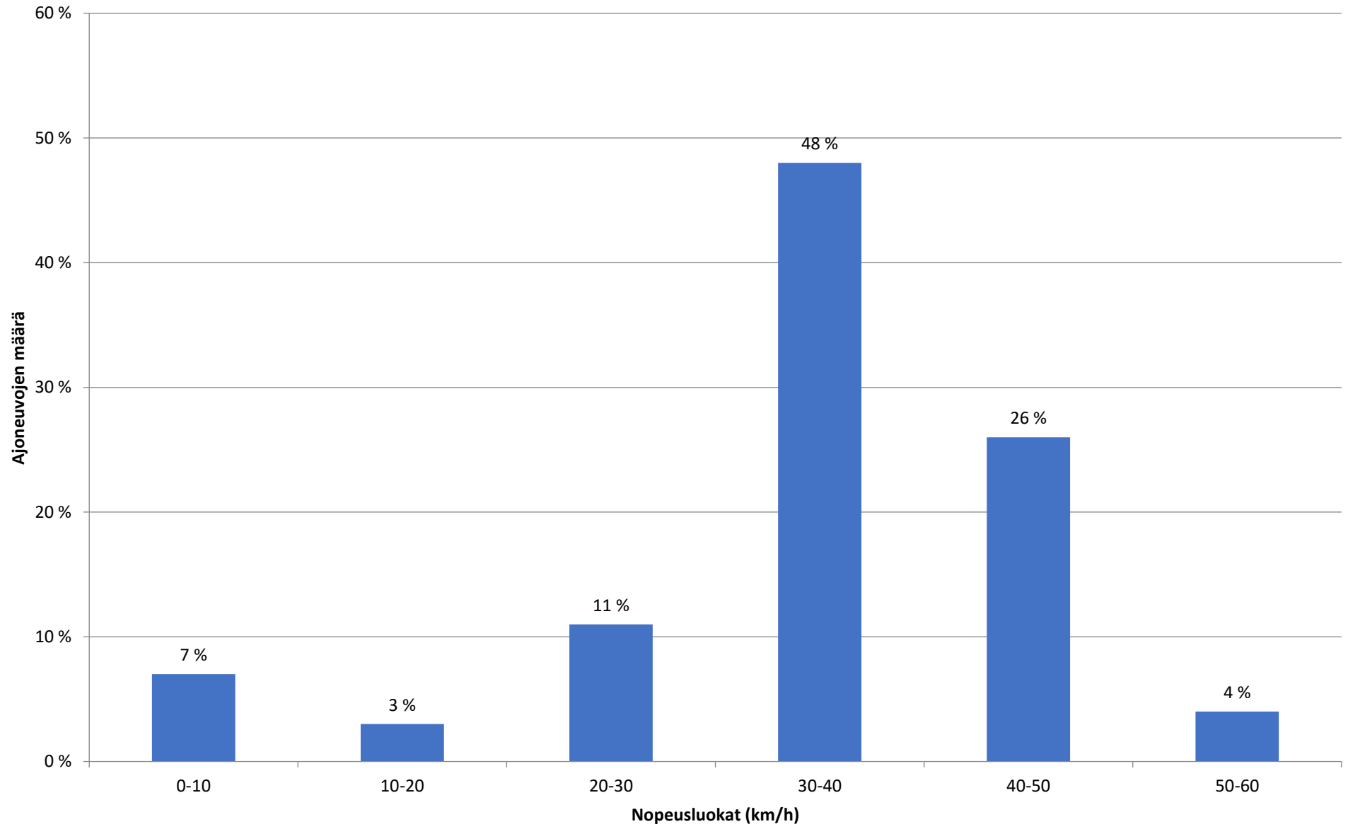
Nopeusjakauma - Koko mittaus - Piste 5 suunta A
