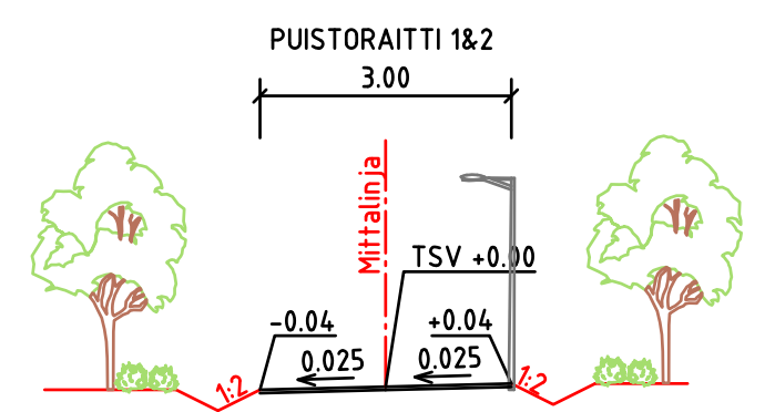
TYYPPIPOIKKILEIKKAUS 1:100
