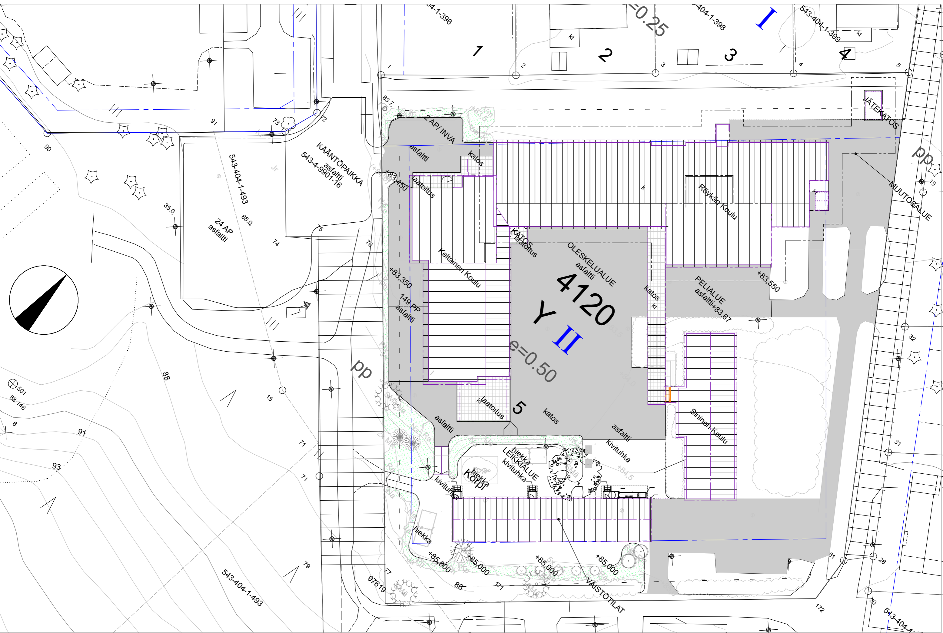
Rökän koulun peruskorjaus, Luonnos 9.2.2021, Asemapiirustus 1:500
