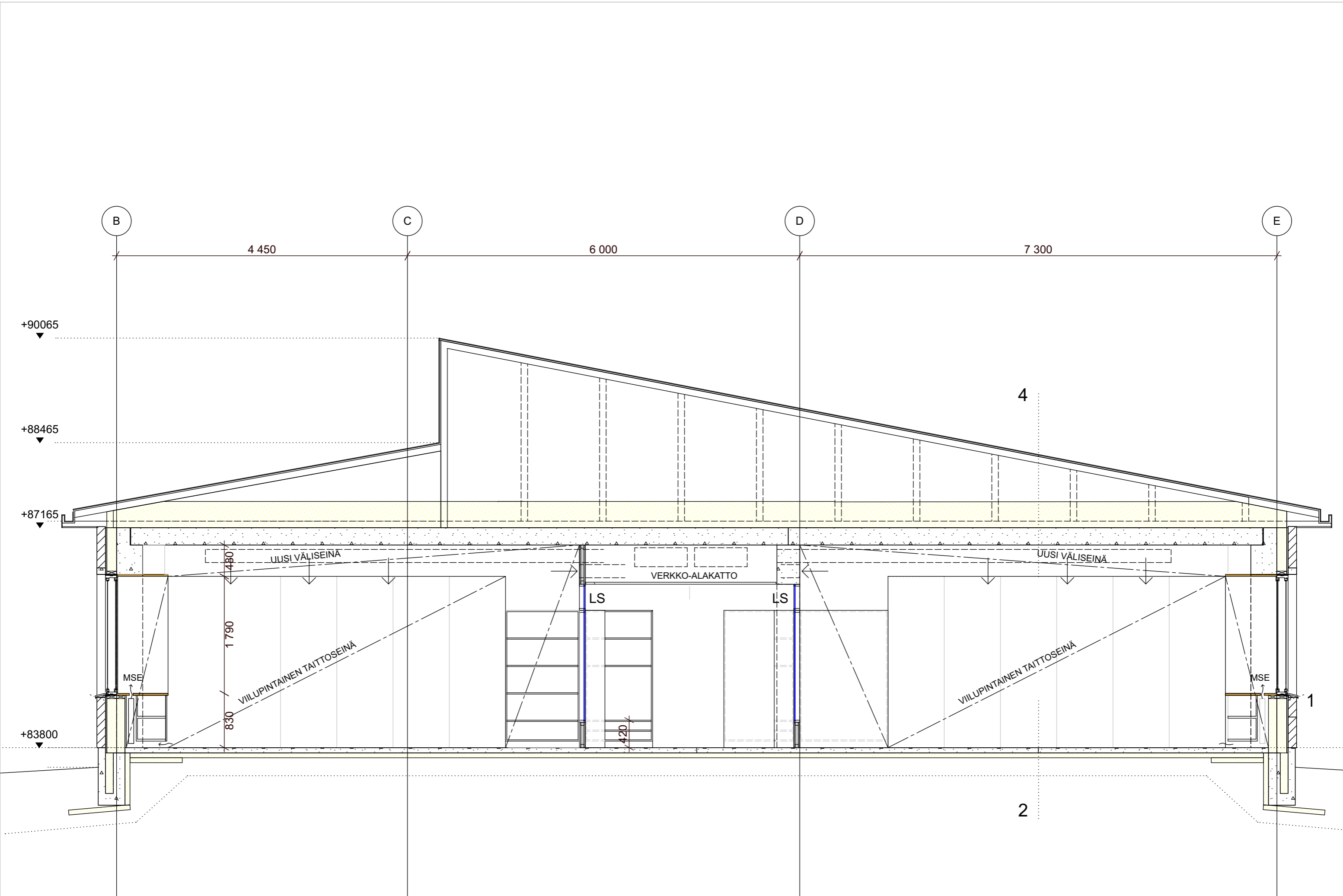
Röykän koulun peruskorjaus, Luonnos 9.2.2021, Leikkaus 1:50
