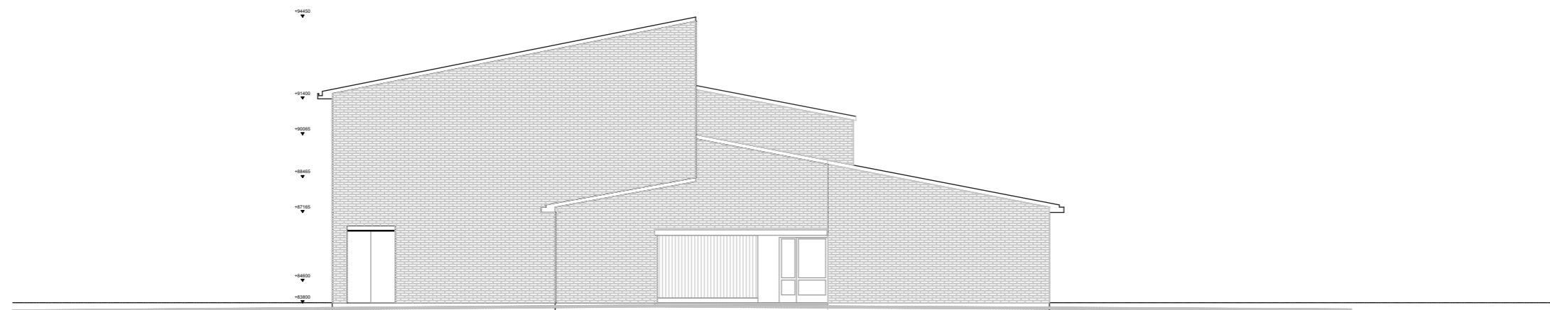
JULKISIVU KOILLISEEN 1:200
