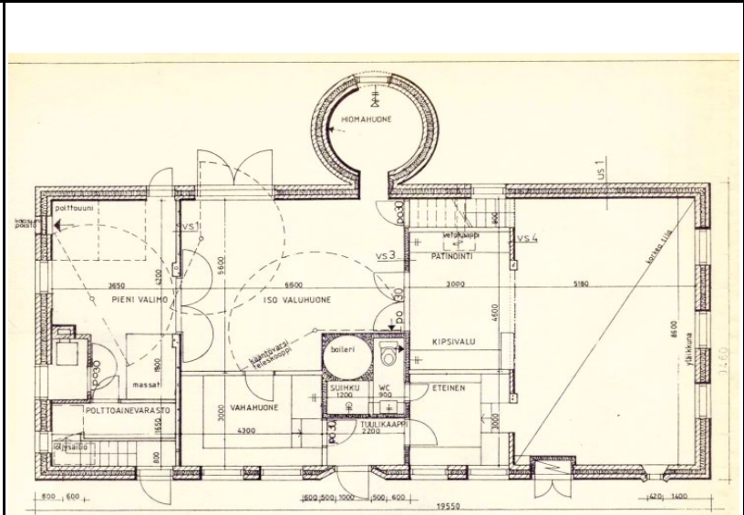
Ateljeen (2) 1. kerroksen pohjapiirustus (1985).
