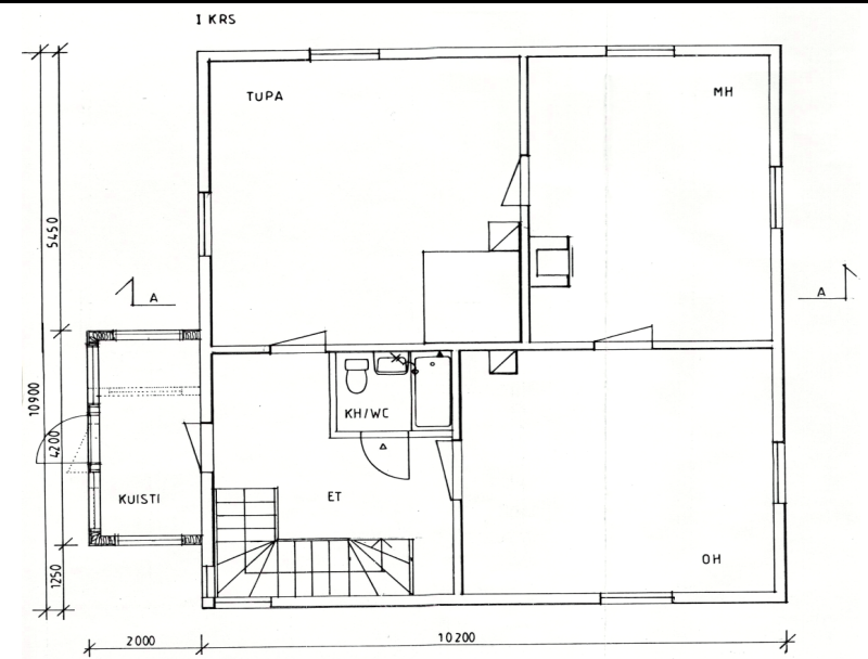
Päärakennuksen 1. krs. pohjapiirustus
